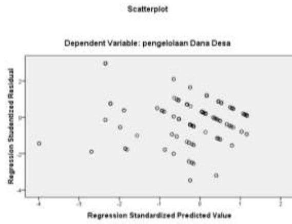
Gambar 3. Uji Heterokedastisitas
