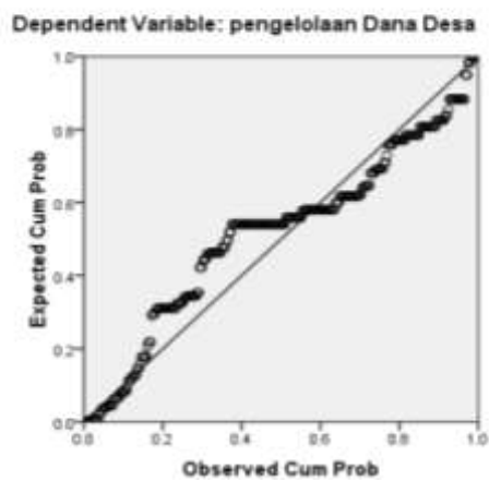
Gambar 2. Uji Normalitas
